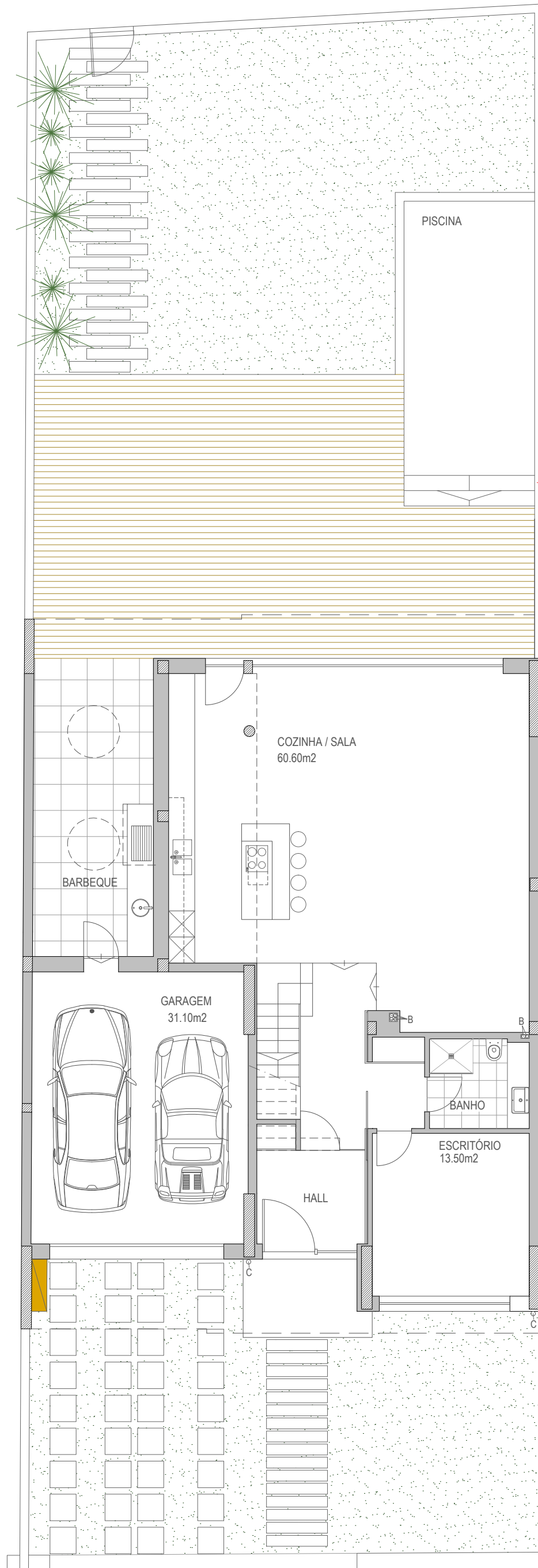
Planta do R/Chão
